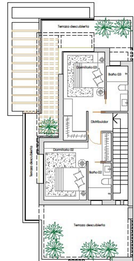
PLANTA PRIMERA
